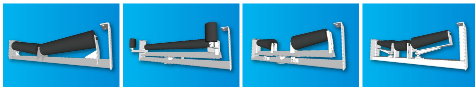
V R型リターンアイドラ VR型
